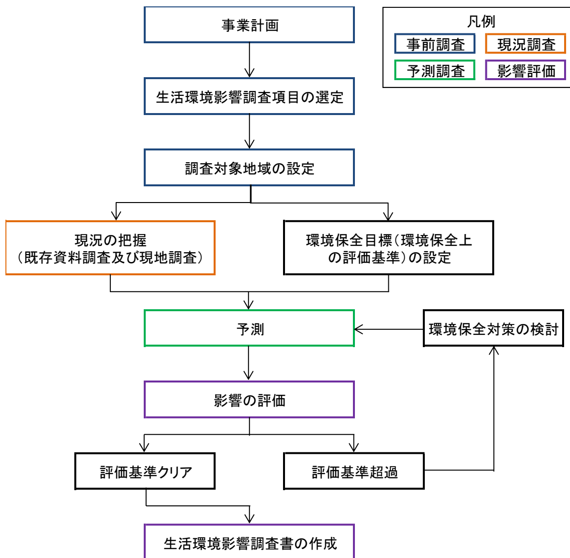
図 3.1-1 生活環境影響調査フロー
